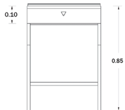
ALZADO FRONTAL
