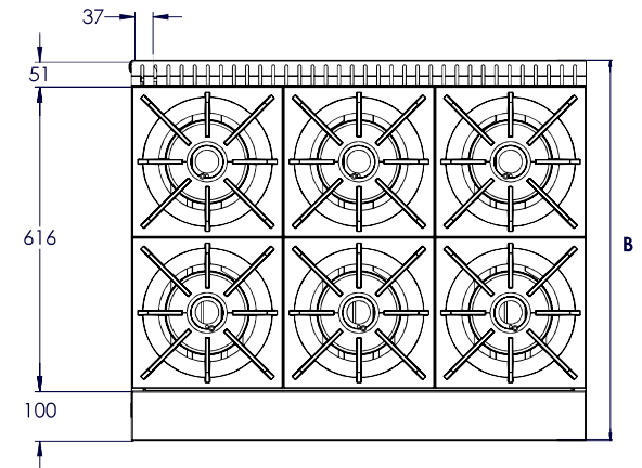
VISTA SUPERIOR
