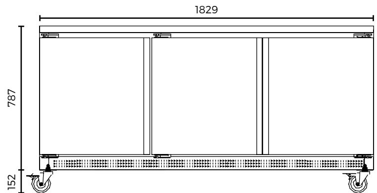
AUTR-72
